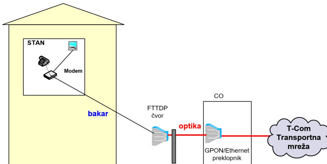
Način realizacije FTTPD koncepta u pristupnoj mreži
